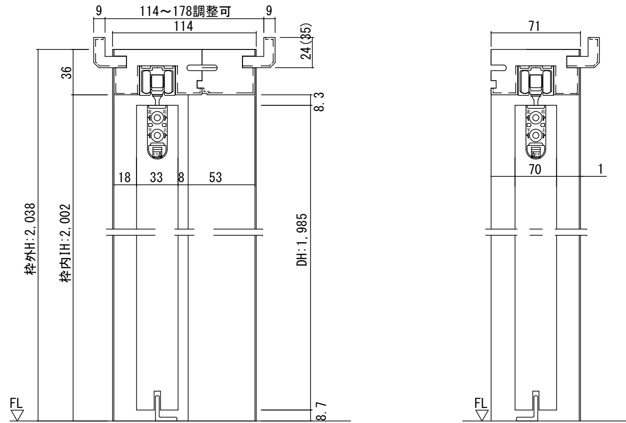
断面図
